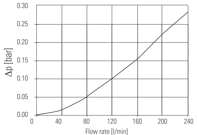
DHP 250 /400
